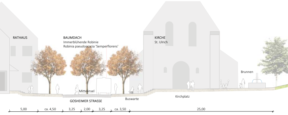
SCHNITT RATHAUS/KIRCHE M 1:100
