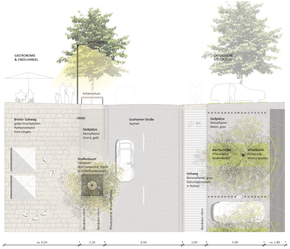
SCHNITT GOSHEIMER STRASSE M 1:50
