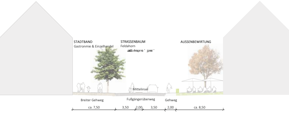
SCHNITT QUERUNG KREISVERKEHR M 1:100
